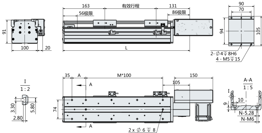
电机左折-L
