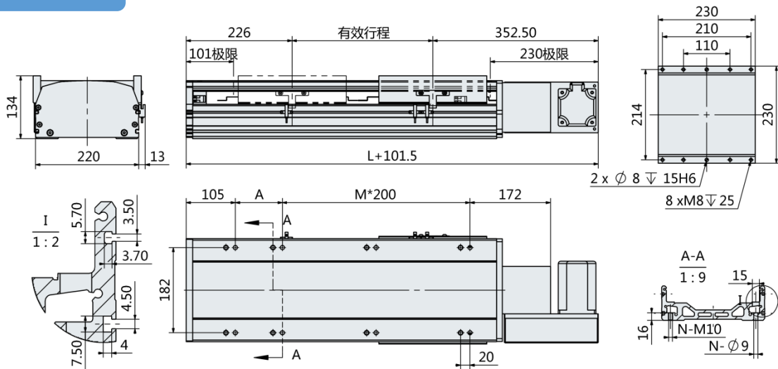
马达右折-R
