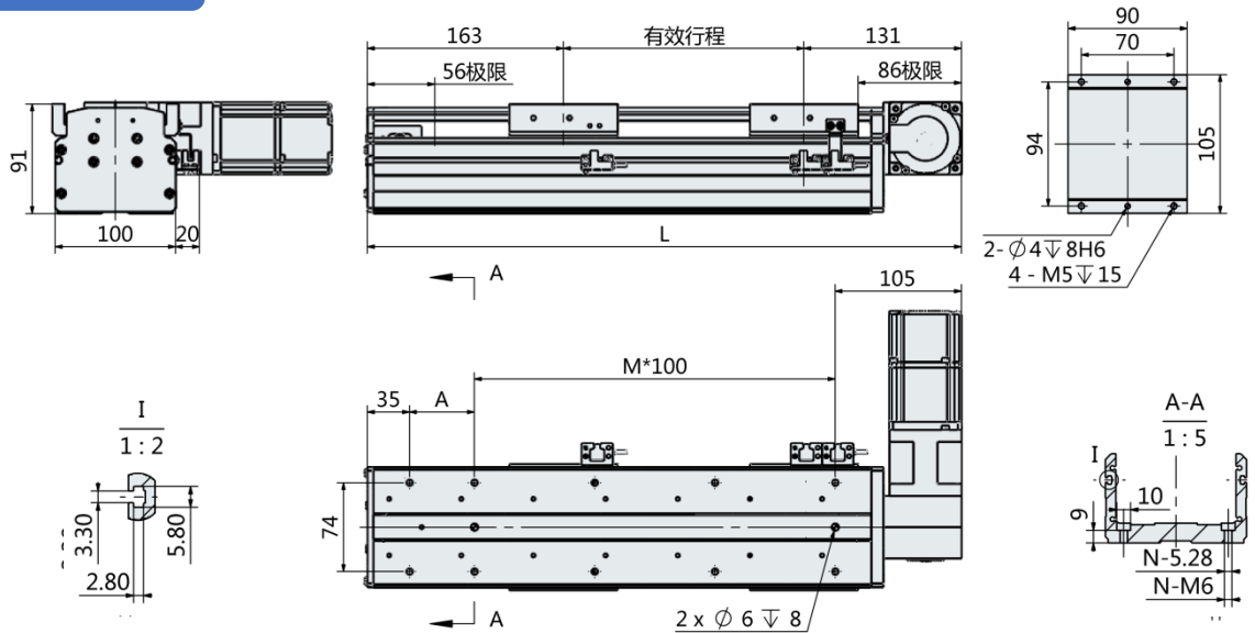
电机直接右折-RT
