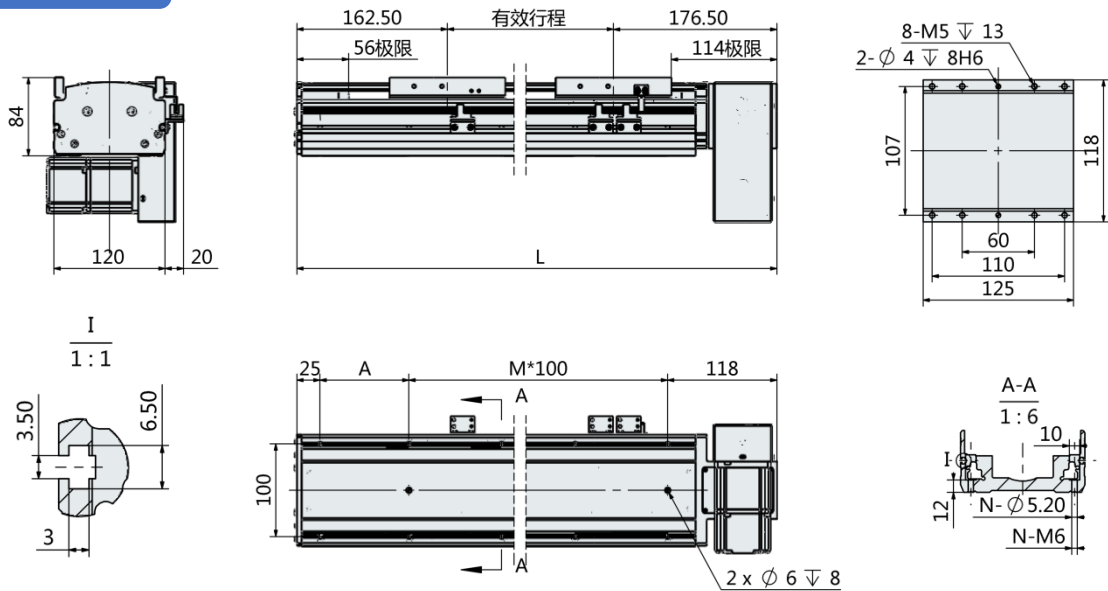
电机左下折-LD
