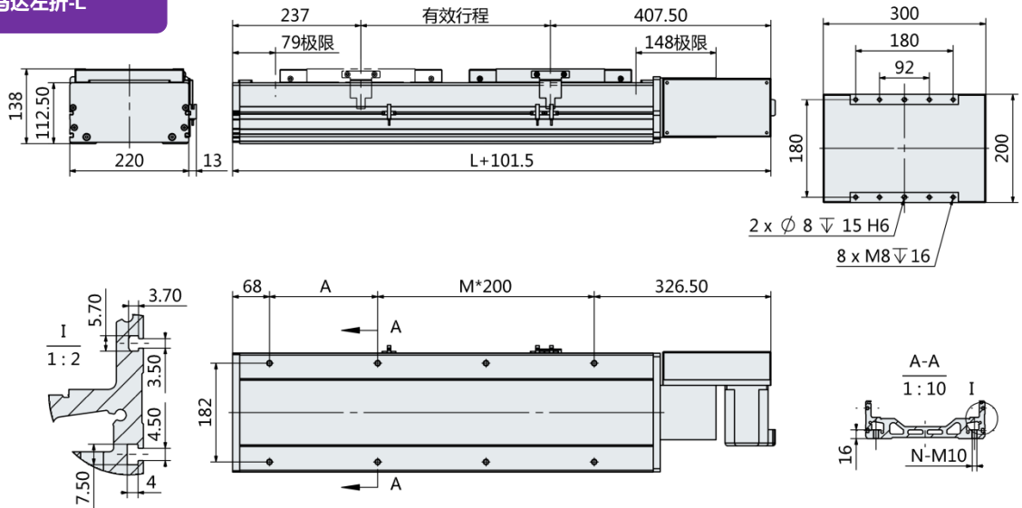
马达左折-L
