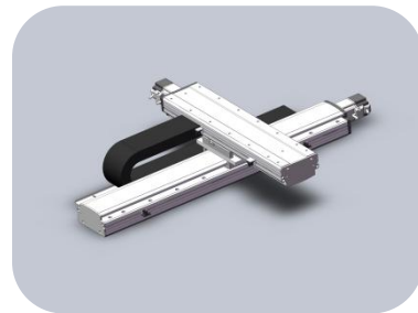
2 XY两轴十字 (Y轴本体移动)
