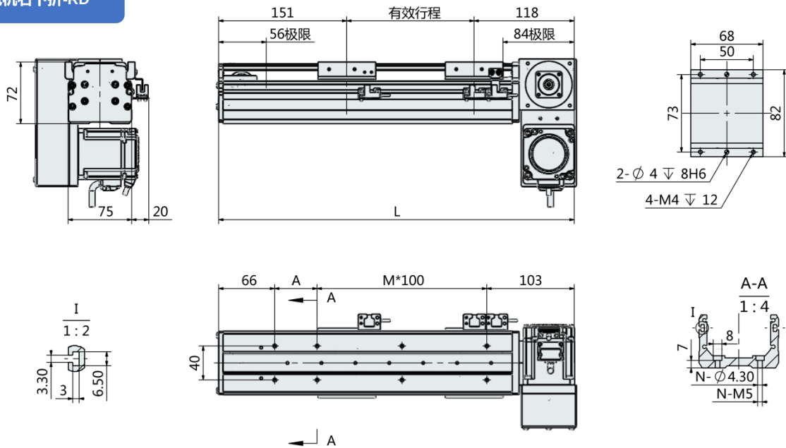
电机右下折-RD
