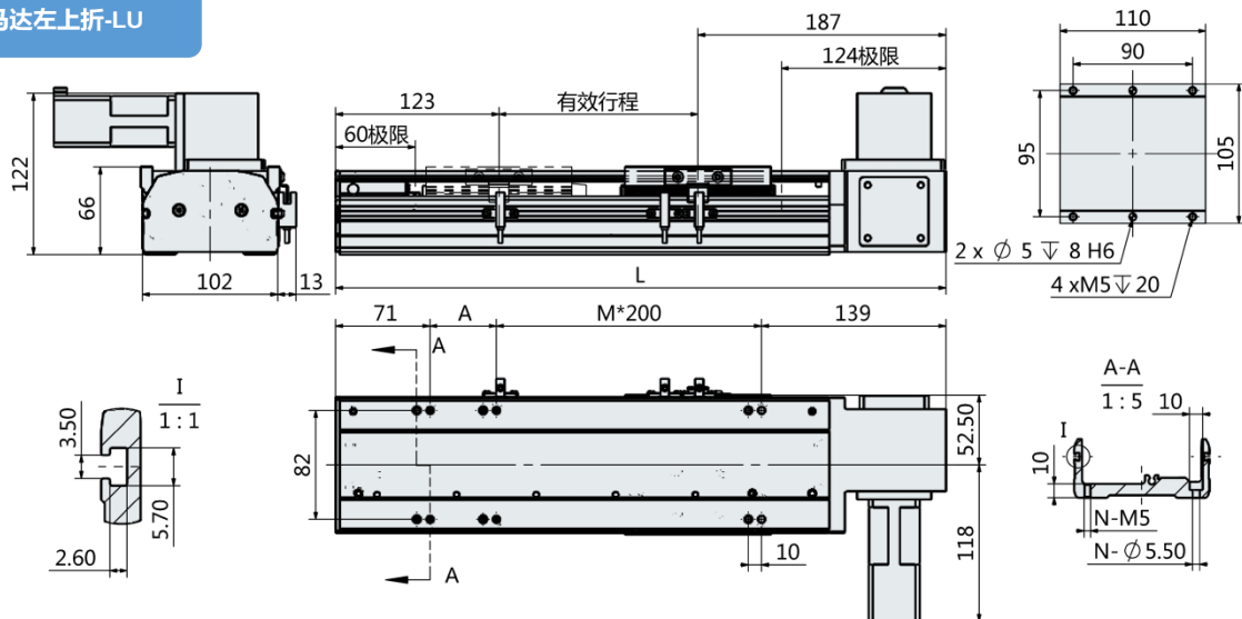
马达左上折-LU
