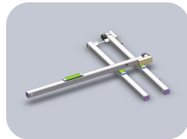
13 XY两轴悬臂 (皮带同动)
