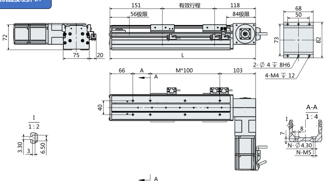
电机直接左折-LT
