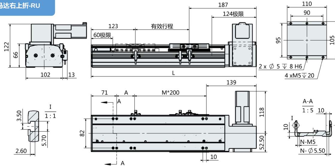
马达右上折-RU
