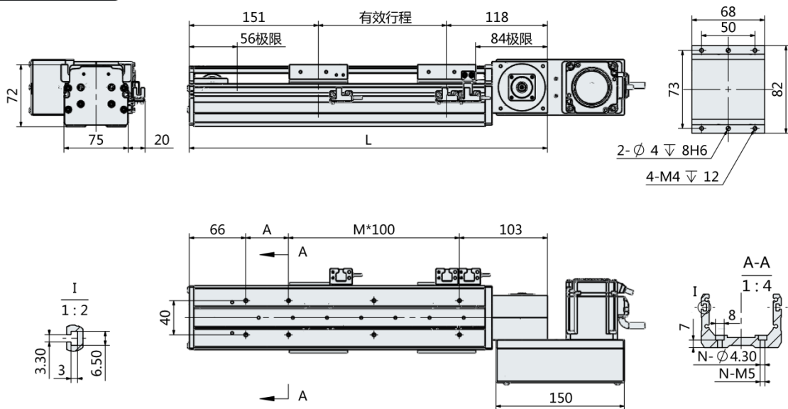
电机右折-R
