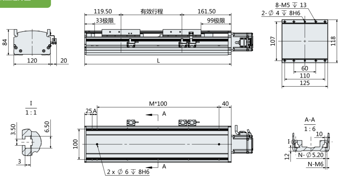
电机直连外置-BC
