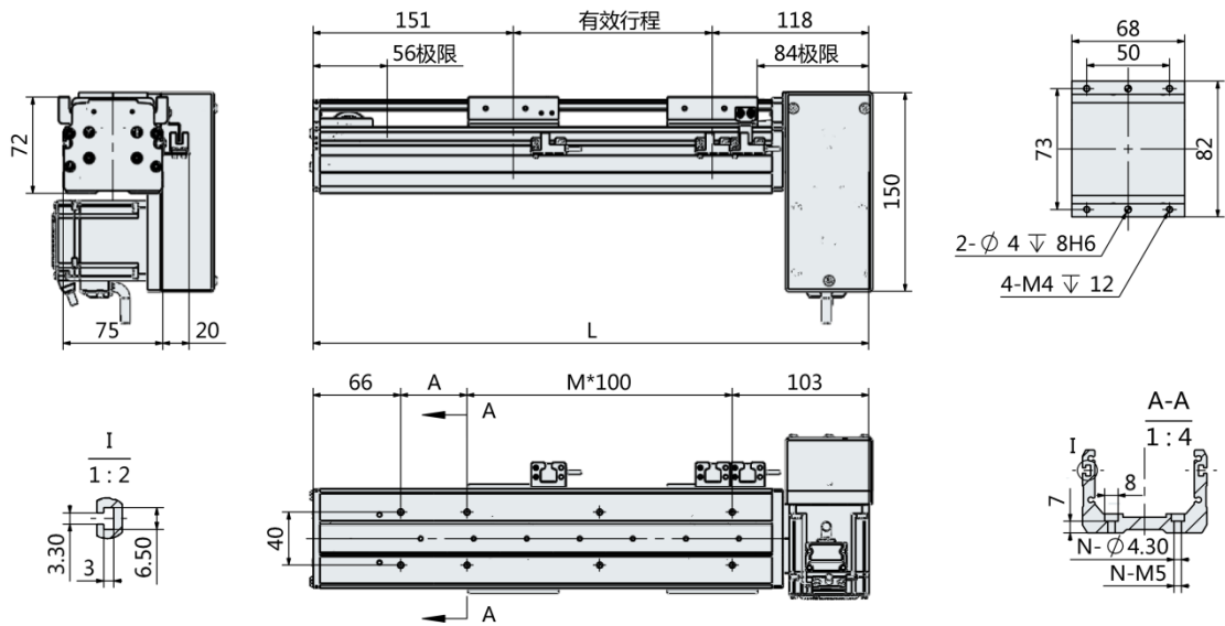
电机左下折-LD
