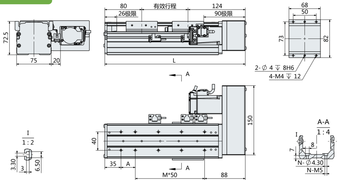
电机右折-BR
