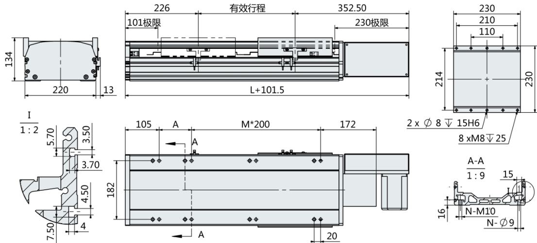
马达左折-L
