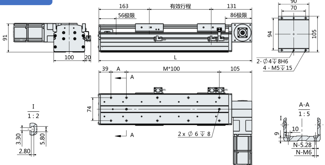
电机直接左折-LT
