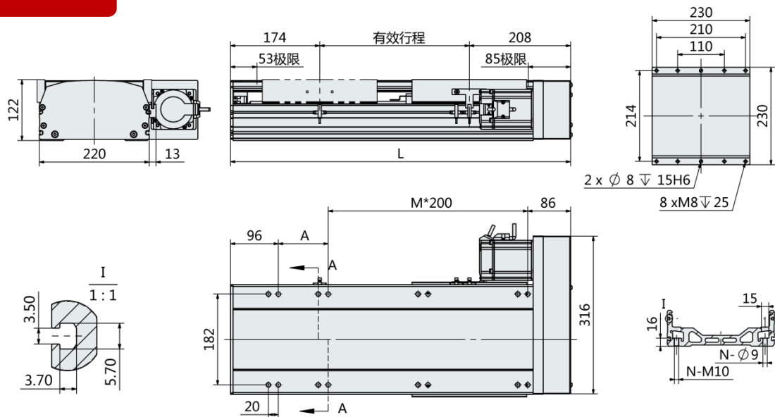
电机右折-BR
