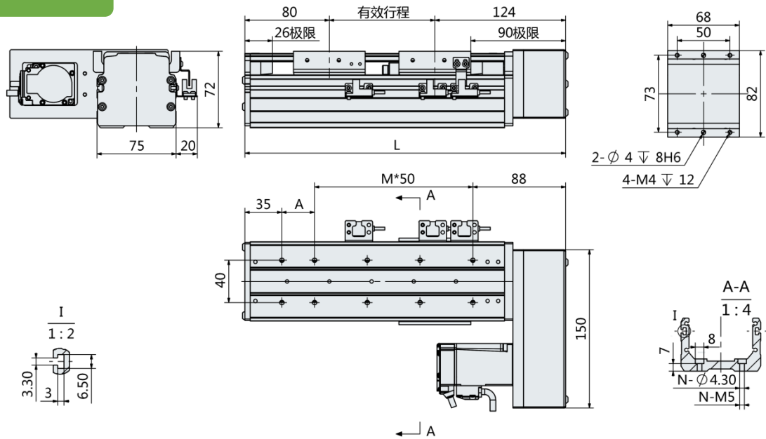
电机左折-BL
