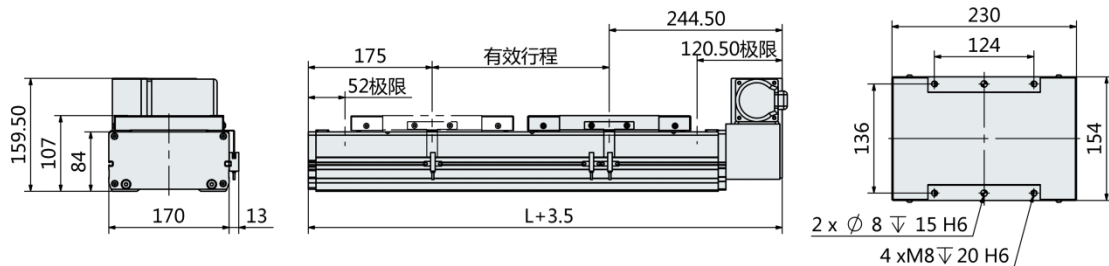
马达右上折-RU
